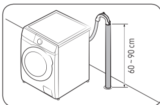
En una tubería de desagüe
